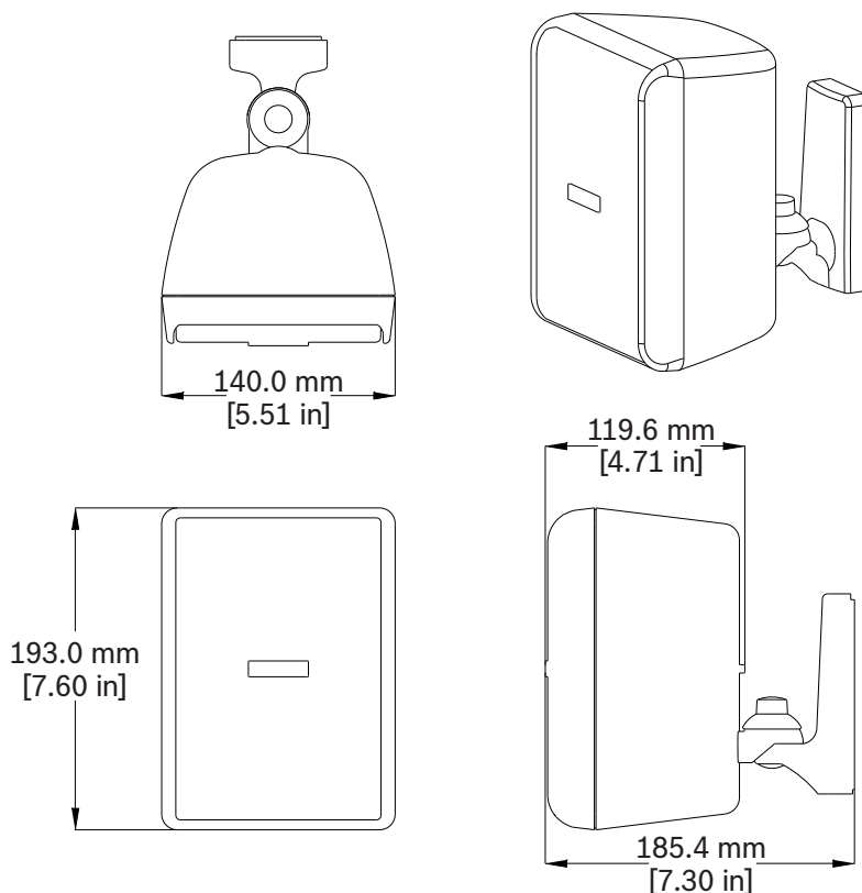
Figure 6.1: LB20-PC40-4/LB20-PC15-4 dimensions
